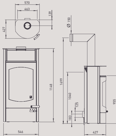
Koko 2.0 mit Speckstein Warmhaltefach
